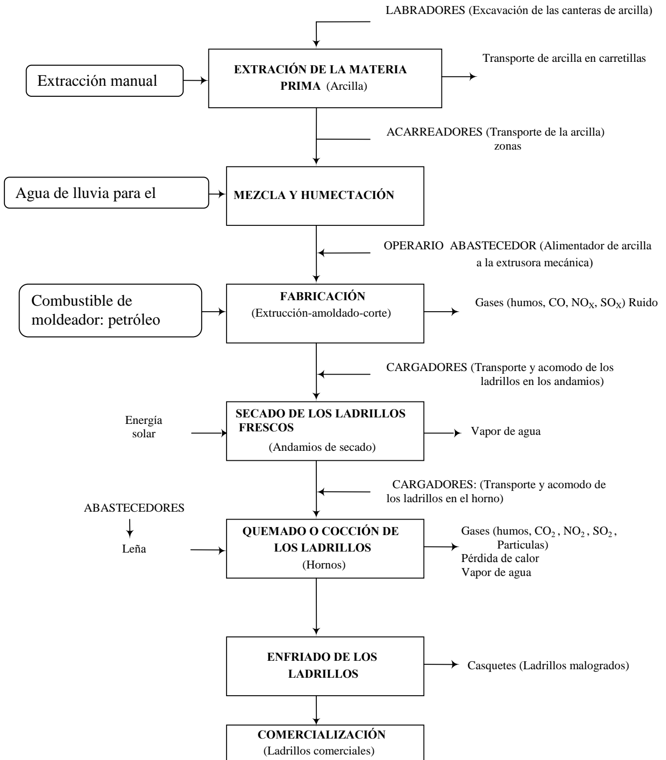
Figura 01: Flujograma de proceso productivo
